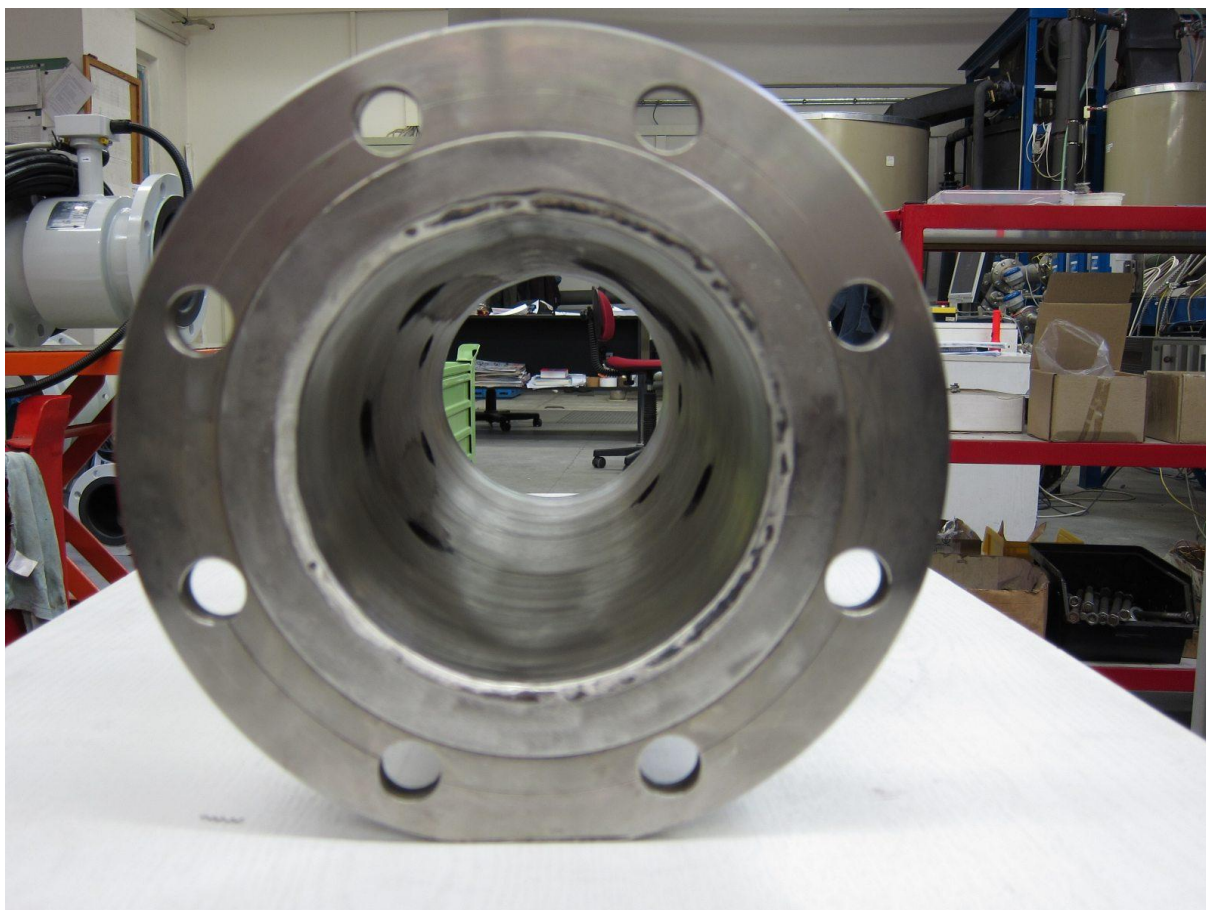
Obr. 3: Pohled na průtočnou část funkčního vzorku s otvory pro ultrazvukové paprsky
