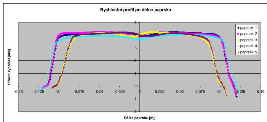
Obr. 1: CFD model prvního návrhu pětipaprskového průtokoměru a rychlostní profily na jednotlivých paprscích získané simulací
